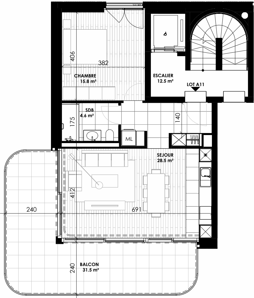
PLAN - 1 : 100
